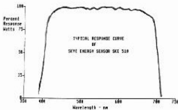
Energie-Sensor SKE 510 (W/m 2 )(mmol/m 2 /s)
