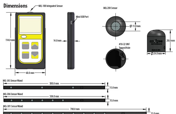
Abmessungen
