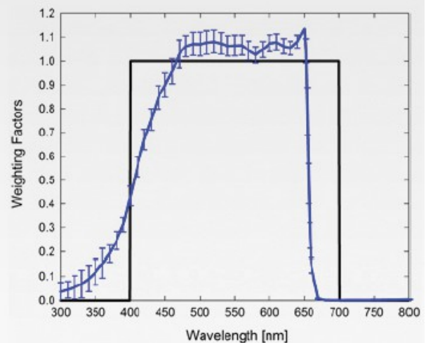
Spektrale Empfindlichkeit
